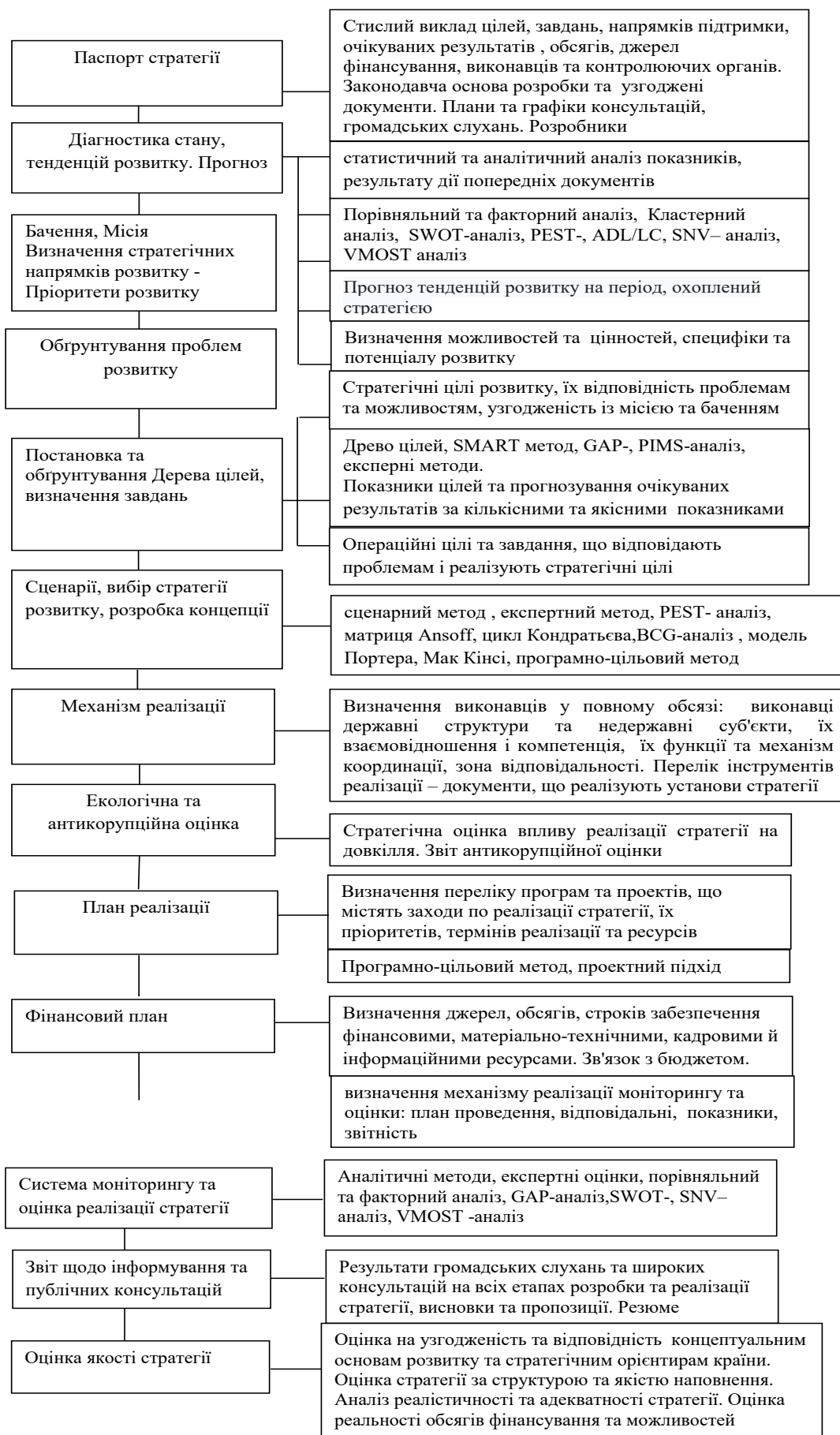
Рис. 1. Загальна структура стратегії соціально-економічного розвитку
