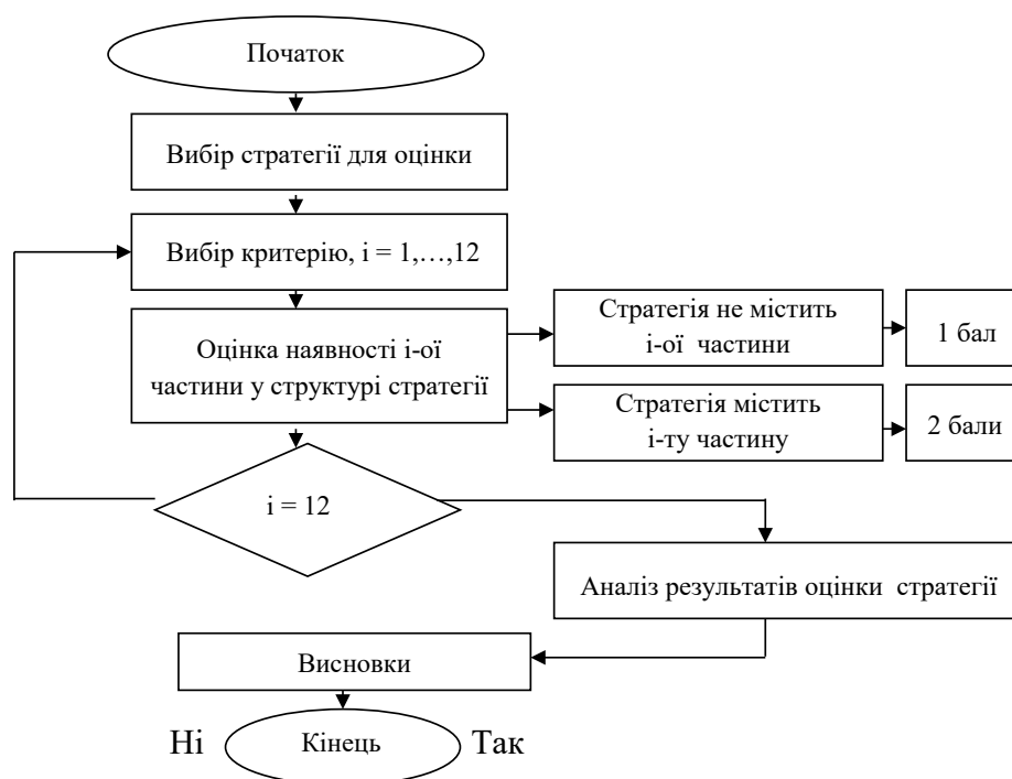
Рис. 3. Алгоритм проведення оцінки стратегій соціально-економічного розвитку за структурою
