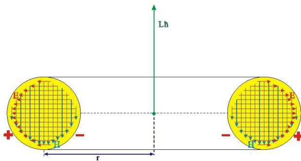
Рис. 3. Будова протона в польовій теорії (поперечний розріз) ( E – постійне електричне поле, H – постійне магнітне поле, жовтим кольором відмічене змінне електромагнітне поле)
